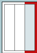
1/3 Seite hoch 40 x 190 Anschnitt-Format 48 x 210 (+3 mm Beschnitt)
